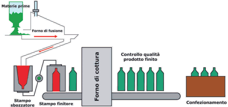
Vetro cavo. Processo produttivo
